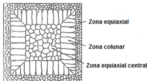
Figura 1. Esquema da estrutura interna de metais solidificados (adaptado de OHNO, 1994)
