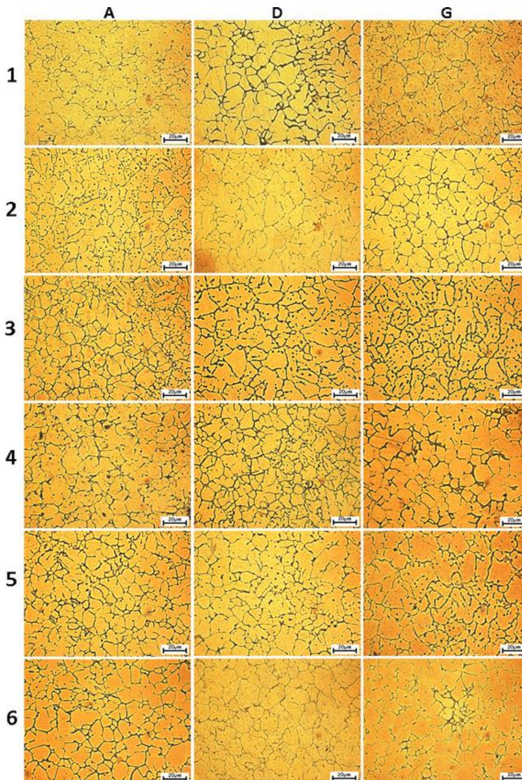
Figura 7. Comparativo das micro-estruturas das amostras
