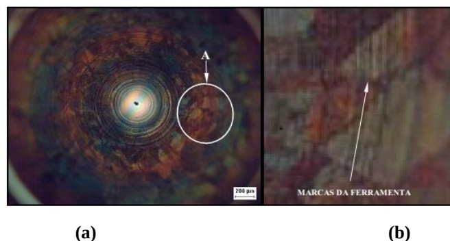
Figura 5. Microscopia óptica de superfície. (a) Contornos dos grãos na cavidade anesférica. Magnificação: 200X. (b) Detalhe A ampliado mostra as marcas da ferramenta no mesmo grão.
