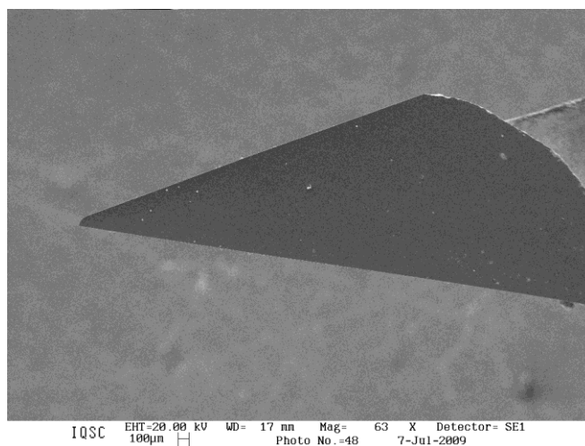
Figura 2. Fotomicrografia feita através da MEV da ferramenta de diamante monocristalino CONTOUR, modelo HCO 10m LGC.
