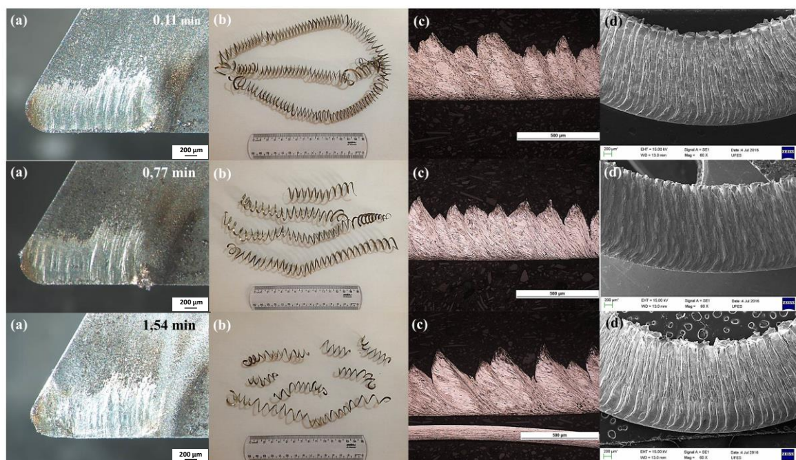
Figura 3. Caracterização dos cavacos de aço inoxidável austenítico produzidos durante o torneamento com a ferramenta de referência. (a) Superfície de saída (Ay) após t_c de 0,11 min; 0,77 min e 1,54 min; (b) cavacos soltos; (c) MO da seção longitudinal dos cavacos; e (d) MEV da superfície livre dos cavacos.
