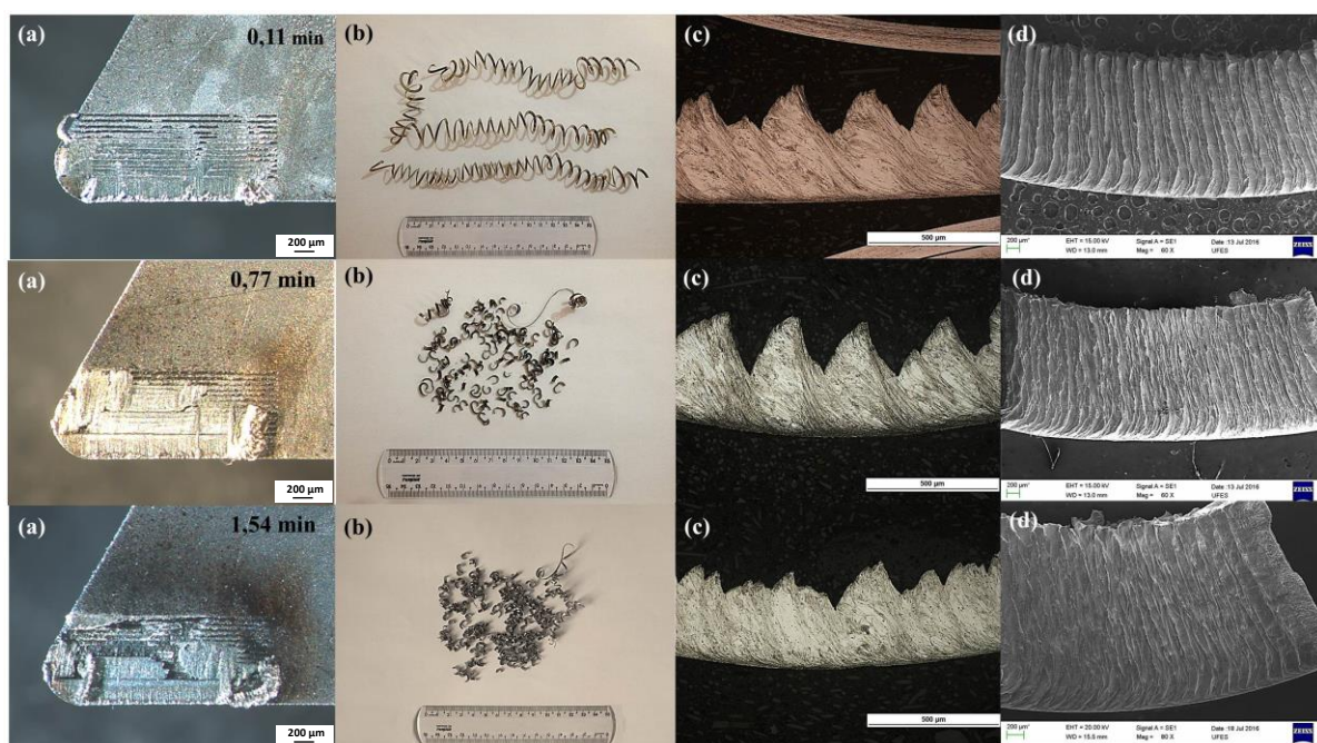
Figura 4. Caracterização dos cavacos de aço inoxidável austenítico produzidos durante o torneamento com a ferramenta texturizada. (a) Superfície de saída (Ay) após t_c de 0,11 min; 0,77 min e 1,54 min; (b) cavacos soltos; (c) MO da seção longitudinal; e (d) MEV da superfície livre do cavaco.
