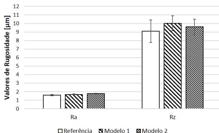
Figura 6. Resultados de rugosidade.
