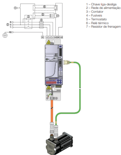
Figura 6. Conexões de potência e controle do servo conversor. (WEG, 2020)
