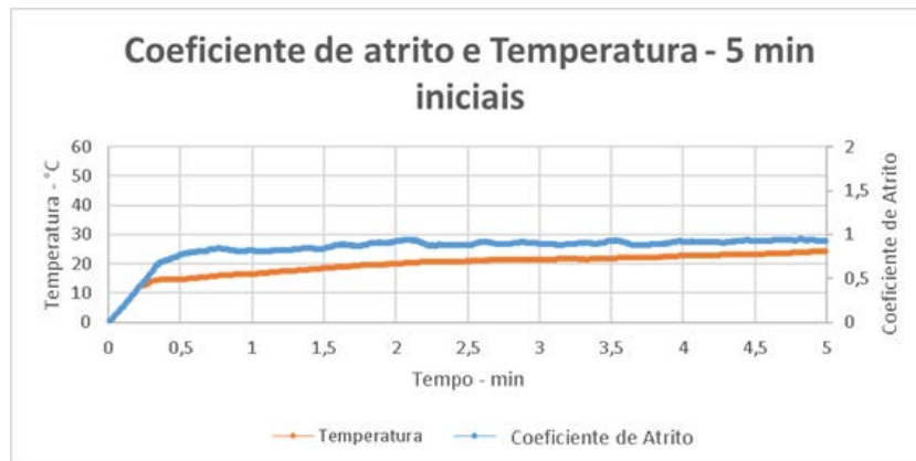
Figura 9 - Coeficiente de atrito e temperaturas para pino de Aço ABNT 1045 normalizado e disco de metal duro sem revestimento com termopar interno, carga de 35 N nos 5 minutos iniciais.
