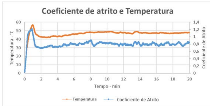
Figura 10 - Coeficiente de atrito e temperaturas para pino de Aço ABNT 1045 normalizado e disco de metal duro revestido com TiN / (Ti,Al)N com termopar extremo, carga de 35 N.
