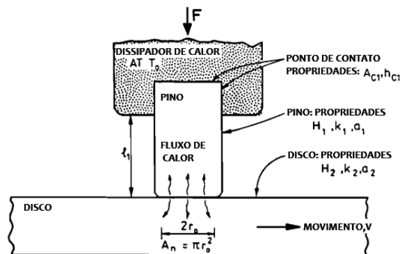
Figura 2 – Configuração padrão para ensaio de pino sobre disco e o fluxo de calor entre os corpos, imagem adaptada (Ashby; Abulawi; Kong, 1991)
