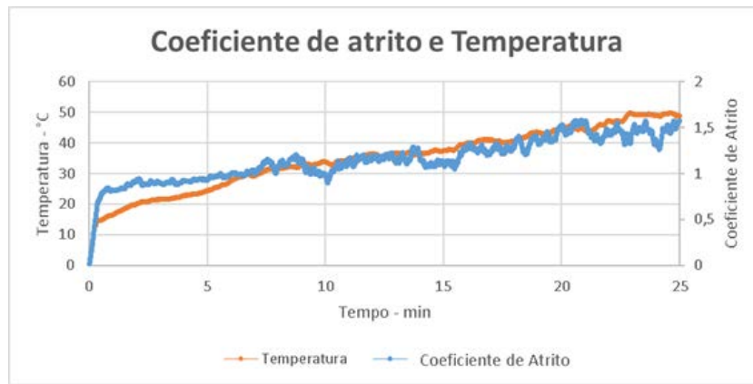
Figura 8 - Coeficiente de atrito e temperaturas para pino de Aço ABNT 1045 normalizado e disco de metal duro sem revestimento com termopar interno, carga de 35 N.
