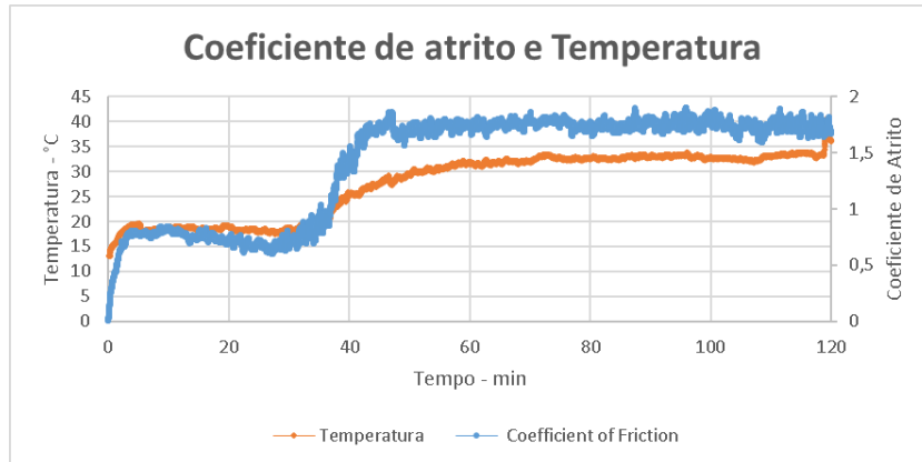
Figura 6 – Coeficiente de atrito e temperaturas para pino de Aço ABNT 1045 normalizado e disco de metal duro P40 sem revestimento com termopar interno e carga de 20N.
