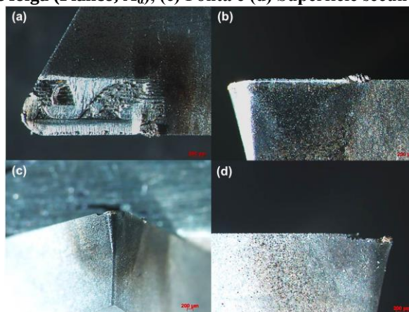
Figura 11. Ferramenta texturizada após o tempo de corte de 3,30 min. (a) Superfície de saída ( A_\gamma ), (b) Superfície principal de folga (Flanco, A_\alpha ), (c) Ponta e (d) Superfície secundária de folga ( A'_\alpha ).
