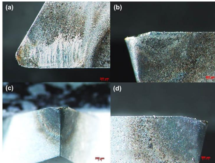
Figura 5. Ferramenta de referência após tempo de corte de 1,54 min. (a) Superfície de saída ( A_{\gamma} ), (b) Superfície principal de folga (Flanco, A_{\alpha} ), (c) Ponta e (d) Superfície secundária de folga ( A'_{\alpha} ).
