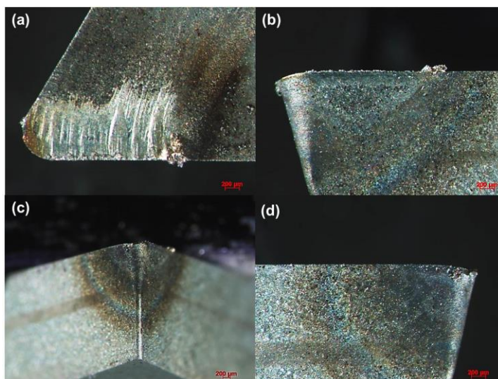
Figura 4. Ferramenta de referência após tempo de corte de 0,77 min. (a) Superfície de saída ( A_{\gamma} ), (b) Superfície principal de folga (Flanco, A_{\alpha} ), (c) Ponta e (d) Superfície secundária de folga ( A'_{\alpha} ).
