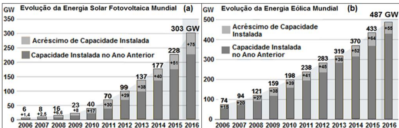
Figura 2. Crescimento das capacidades instaladas mundiais 2006–2016: (a) Solar Fotovoltaica; (b) Eólica, segundo REN21 (2017) (Adaptado).
