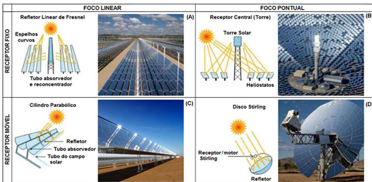
Figura 4. Tecnologias CSP: (A) Refletor Linear de Fresnel; (B) Torre Solar com Receptor Central; (C) Cilindros Parabólicos; (D) Discos de Stirling, segundo TOLMASQUIM (2016) (Adaptado).
